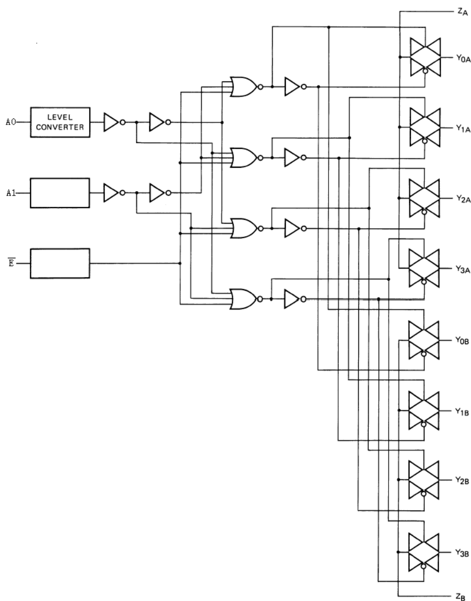
逻辑图
