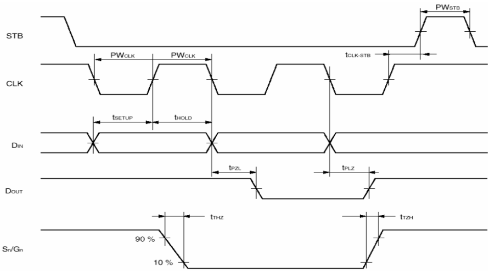
图 4、时序图
