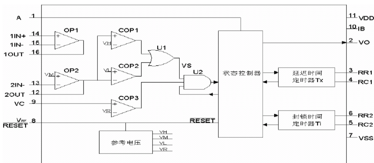
图 1 GS0001 内部结构框图
