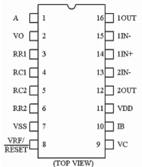
图2 脚位图
