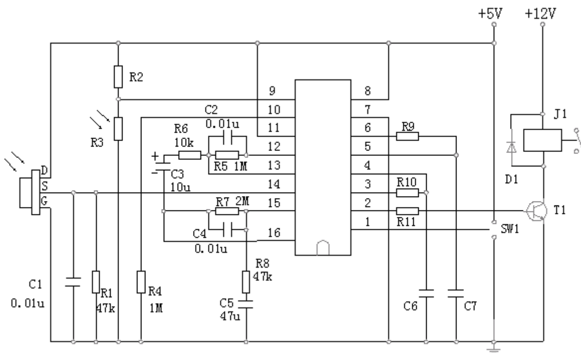
图5 GS0001典型应用图
