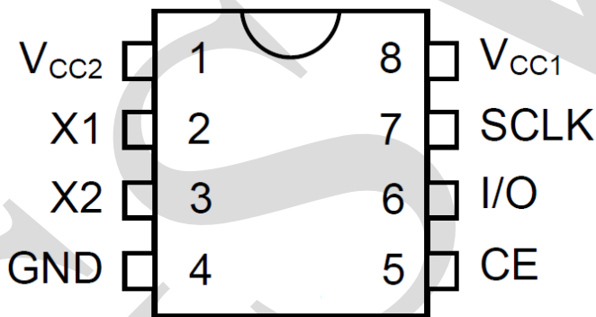
图 3、引脚图（DIP8）
