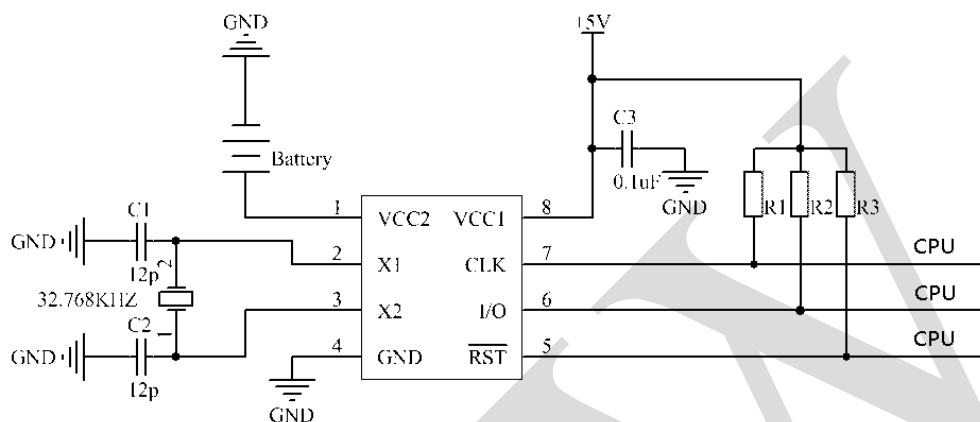
图 12、典型应用图
