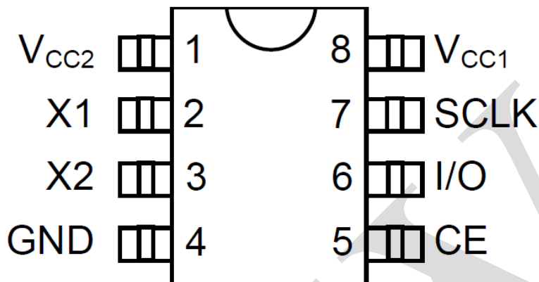
图 2、引脚图（SOP8）
