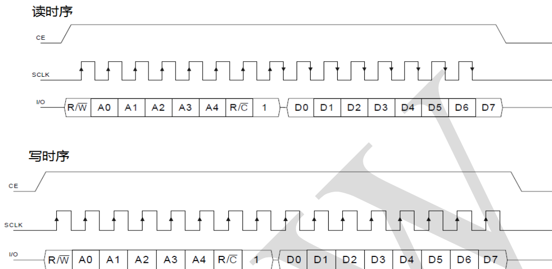
图 8、读写时序
