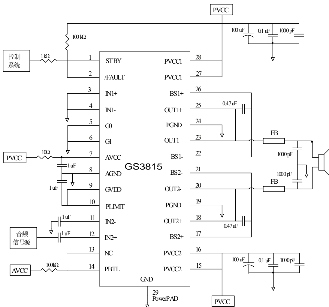
单端输入，PBTL 输出
