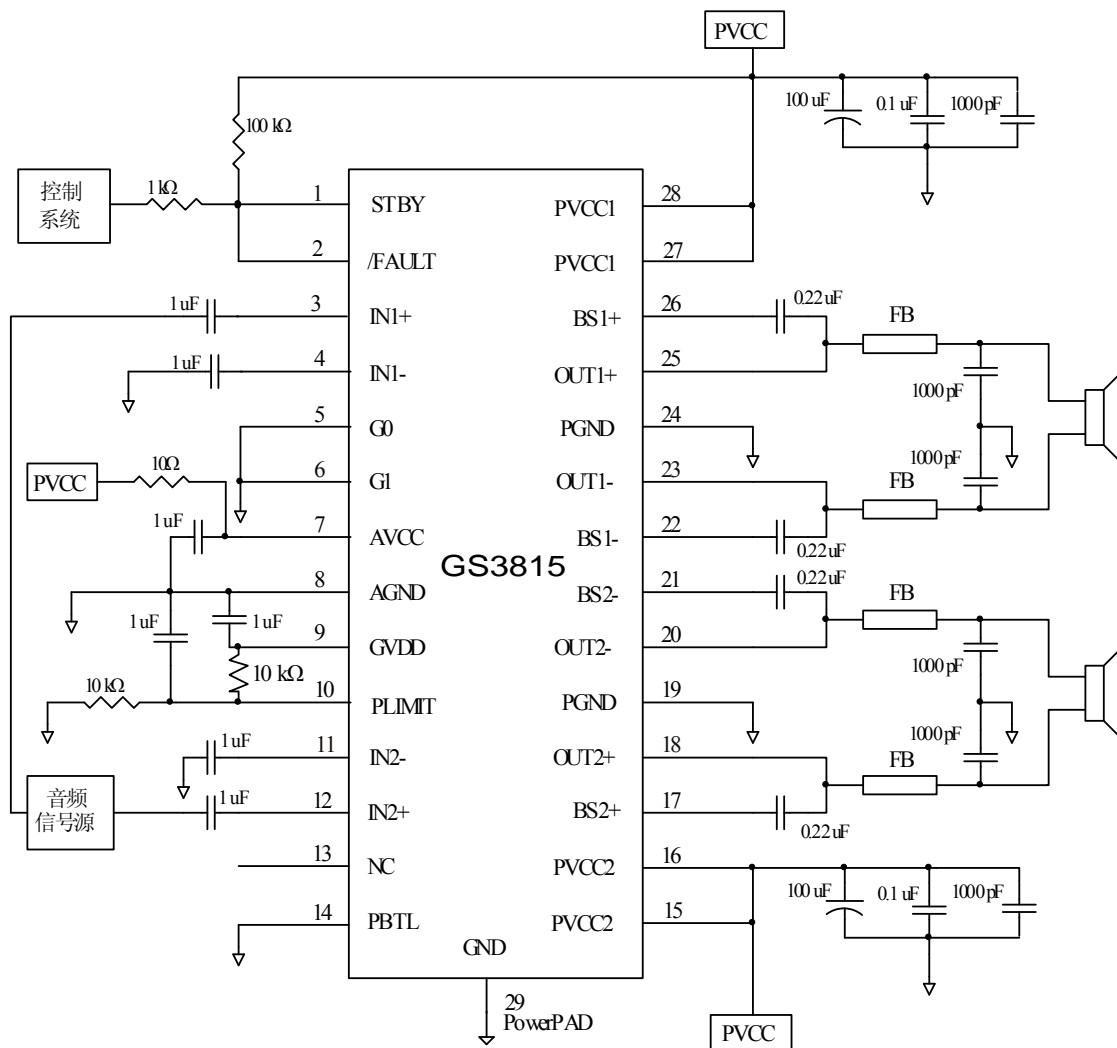
单端输入，BTL 输出
