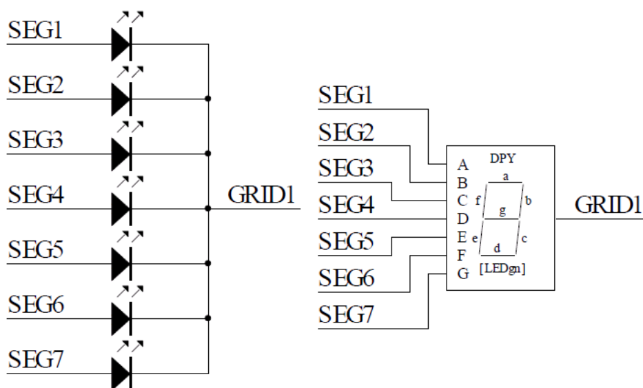
图 5、共阴数码管连接图
