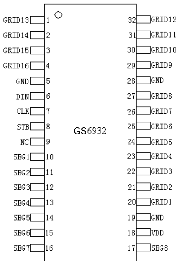
图 1、GS6932 引脚排列图
