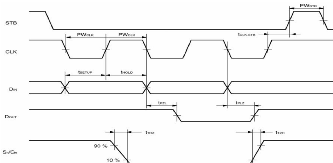
图 2、时序图
