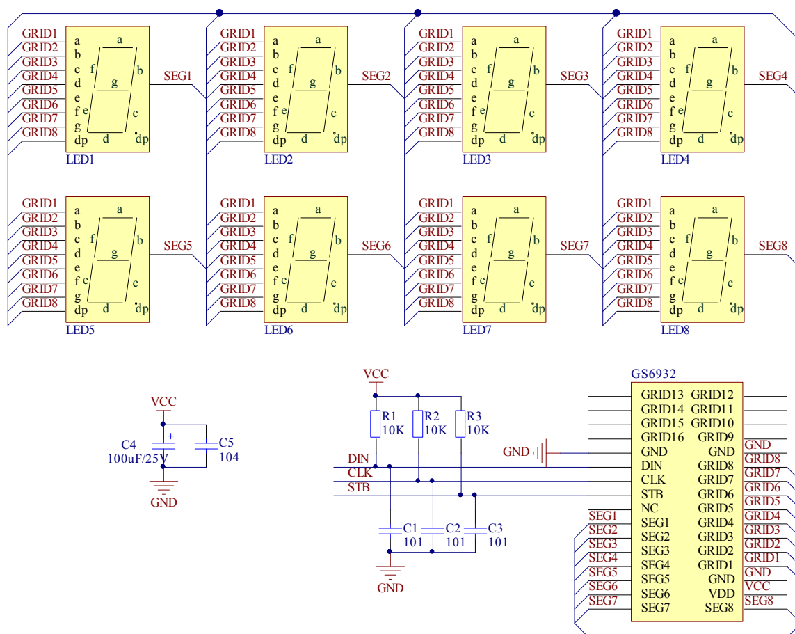
图 12、GS6932 驱动共阳数码管原理图
