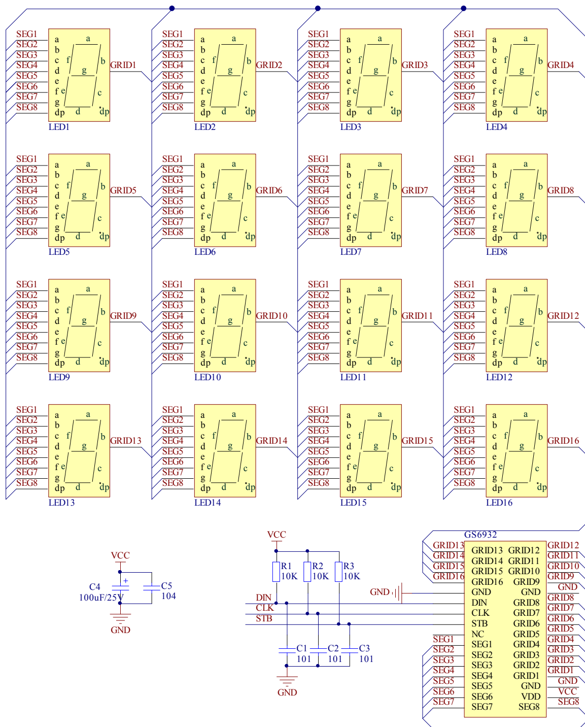
图 11、GS6932 驱动共阴数码管原理图
